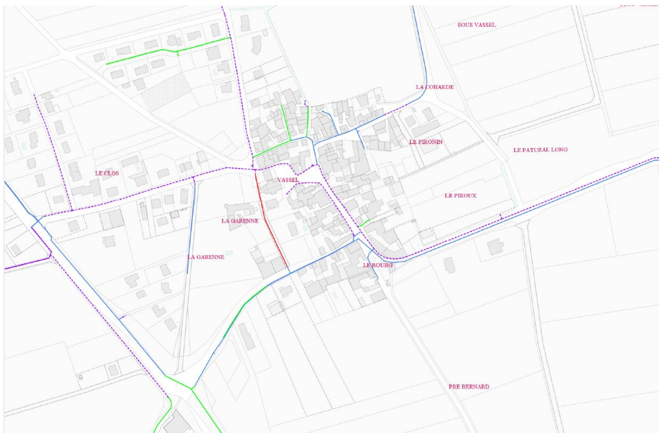
PLAN DU RESEAU D'EAU POTABLE (EN SOUS-TERRAIN)
